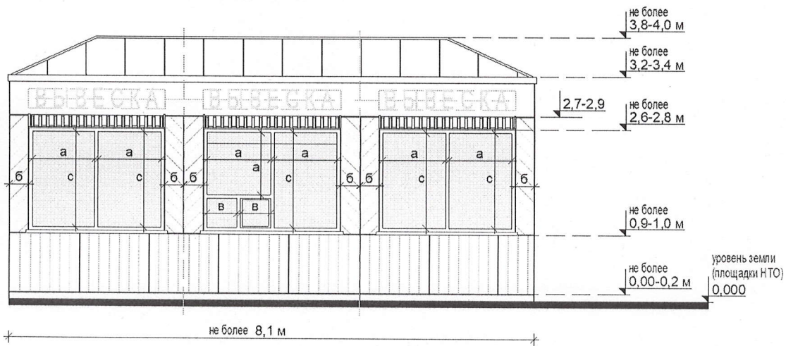
схема с максимальными размерами:
