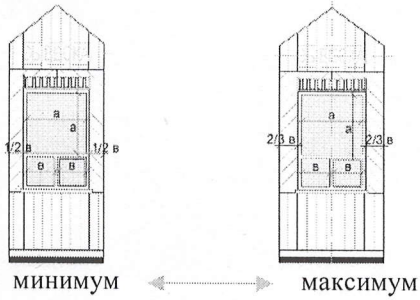
схема допустимого увеличения простенков:
