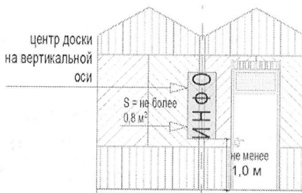
фасад со служебным входом:
