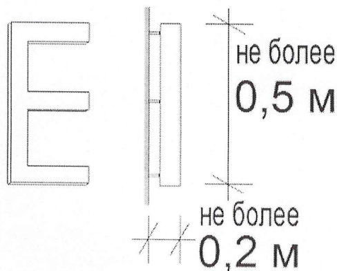
объемные буквы на дистанционных держателях
