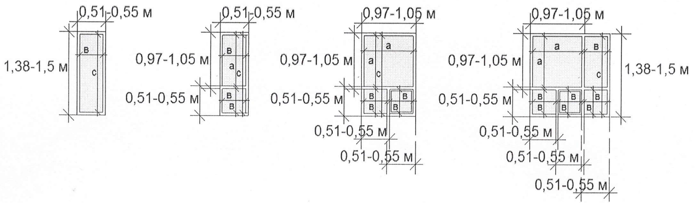
схема допустимого увеличения площади остекления:
