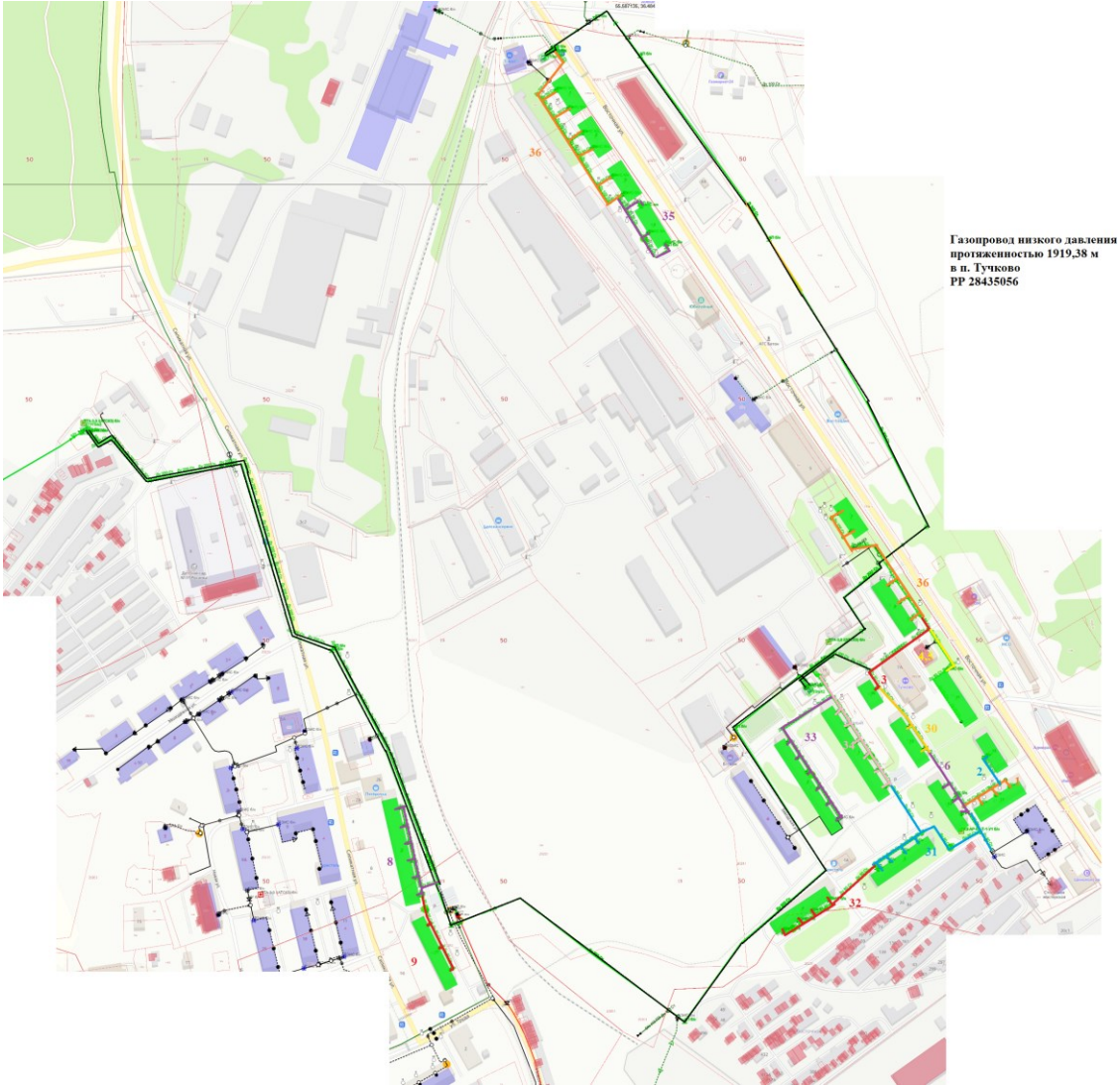
Схема расположения газопровода, расположенного по адресу: Московская область, Рузский муниципальный округ, пгт. Тучково
