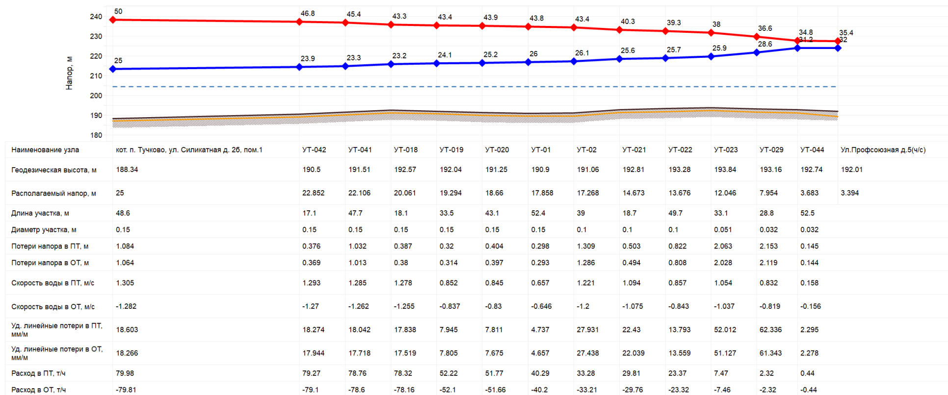
Рисунок 8.4.8 – Пьезометрический график результата электронного моделирования переключения потребителей в зоне действия котельной пгт. Тучково, ул. Силикатная д. 26, пом.1
