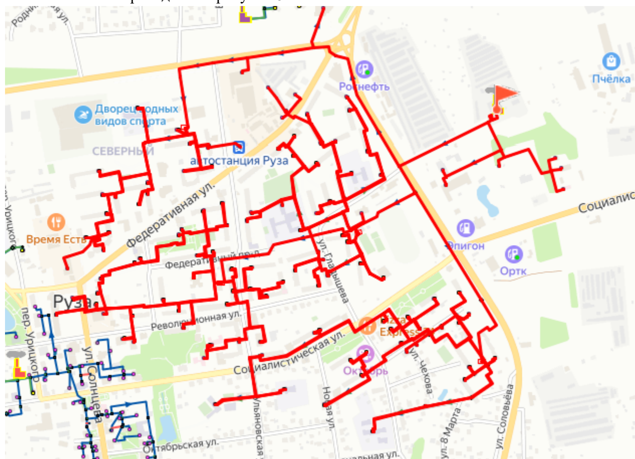
Рисунок 8.4.1 – Зона действия котельной г. Руза, Промзона, уч. №1 в нормальном режиме теплоснабжения
